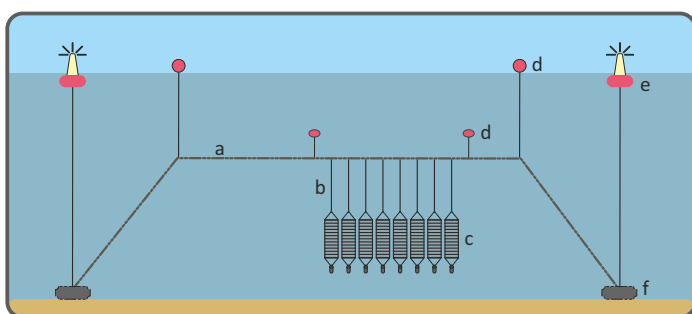
Figura 12. Esquema típico de uma estrutura flutuante com long-lines para produção de ostra em mar-aberto: a. cabo madrep, b. cordas suspensas, c. lanternas, d. flutuadores, e. bóias do assinalamento marítimo, f. poitas e âncoras. Ilustração Paula Gaspar.
